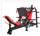
LP-021 Super Leg Press 45° Duplo Dimensão (mm) 2475 x 1790 x 1645 Peso 405kg
