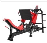
LP-020 Super Leg Press 45° Dimensão (mm) 2450 x 1770 x 1620 Peso 380kg
