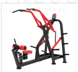
LP-047 Super Lat Machine Dimensão (mm) 2075 x 1445 x 1895 Peso 230kg
