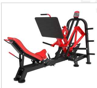
LP-022 Super Leg Press Articulado Dimensão (mm) 2605 x 1605 x 1630 Peso 320kg
